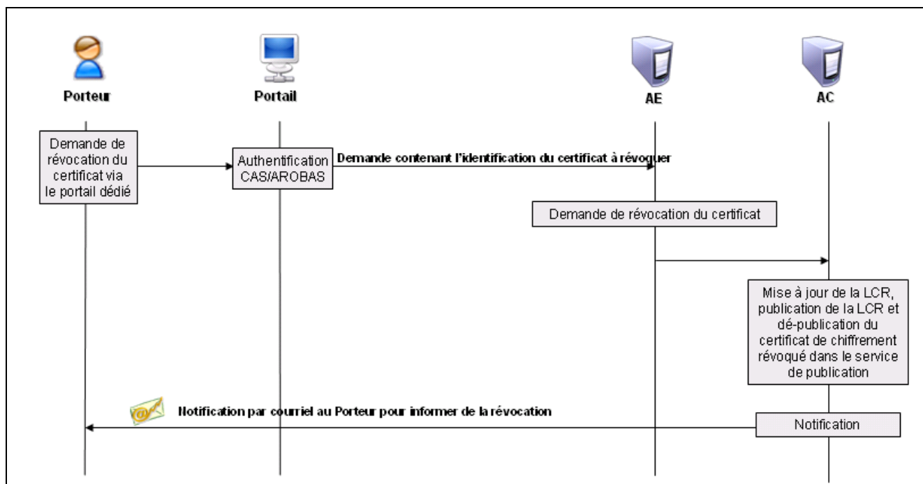
Figure 10 : Processus révocation du certificat de chiffrement par le Porteur via le portail
