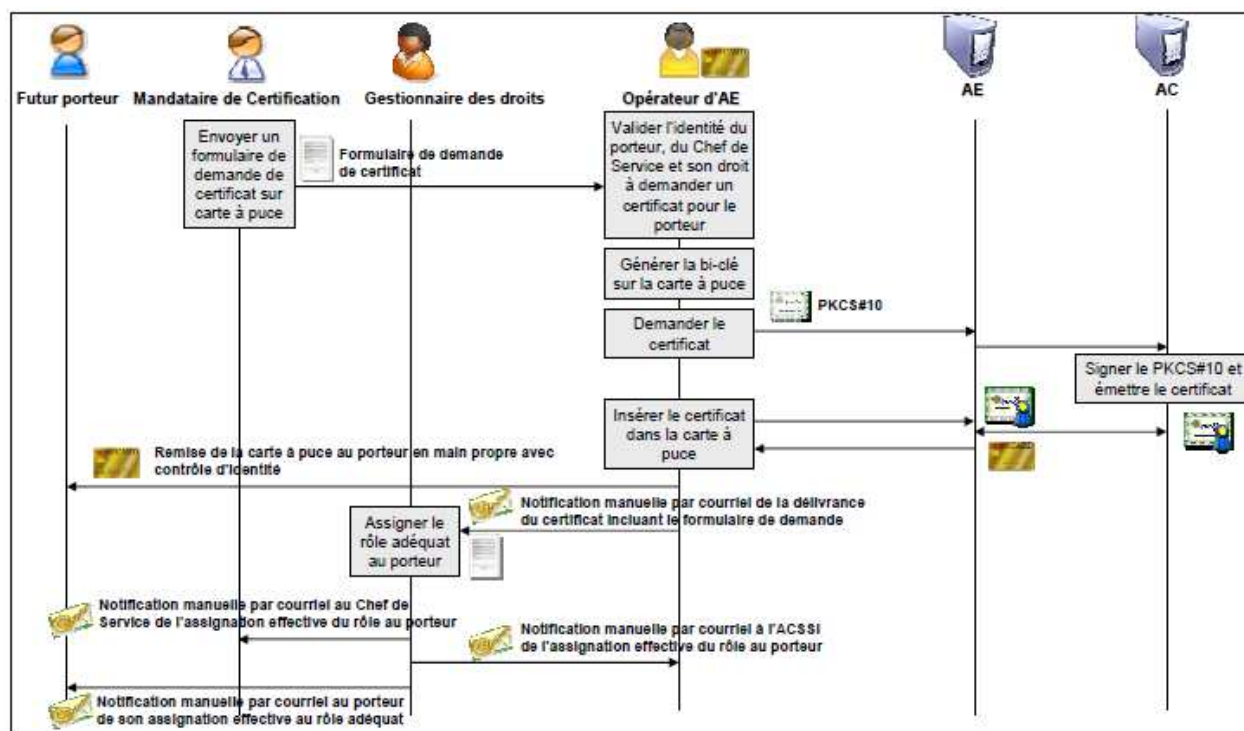
Figure 3 : Processus d'une demande d'un certificat de gabarit « authentification forte agent »
